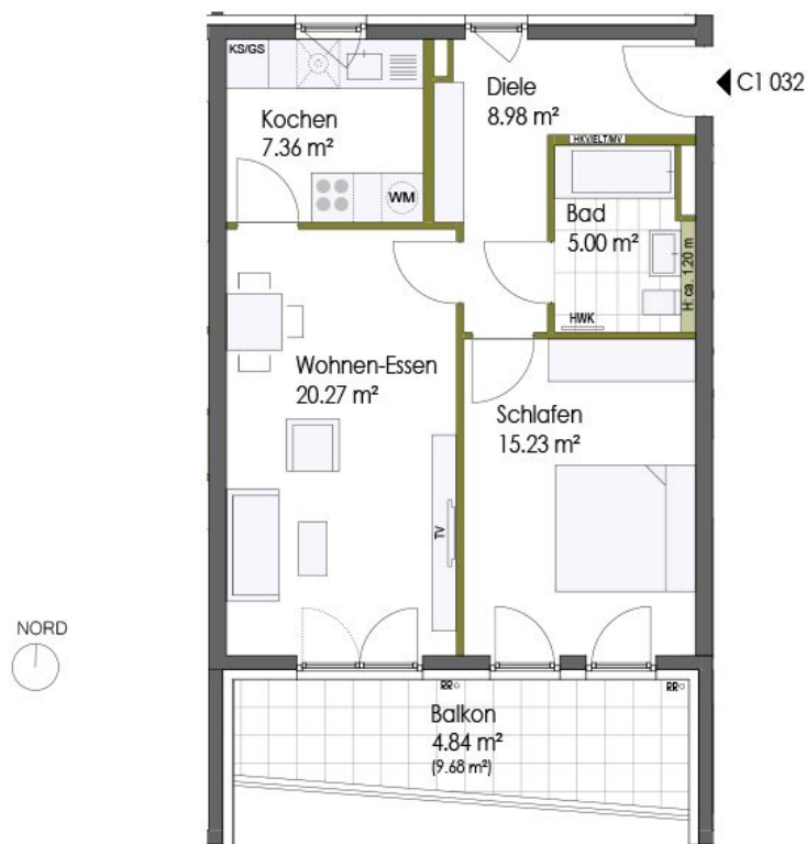
Grundrissplan einer 2-Zimmer-Wohnung mit Balkon
